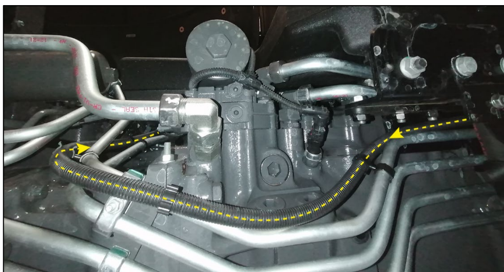
Vista de baixo do veículo
