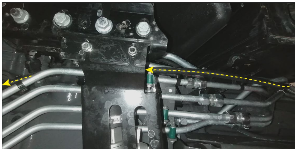
Vista de baixo do veículo
