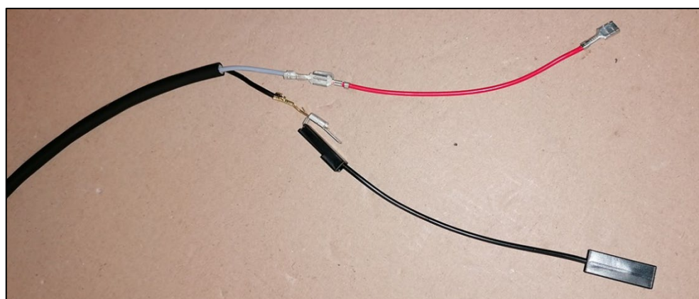
Extensor do chicote de cabos para a tomada de 3 polos
