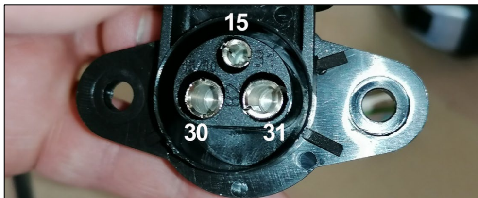
Atribuição dos terminais da tomada de 3 polos
