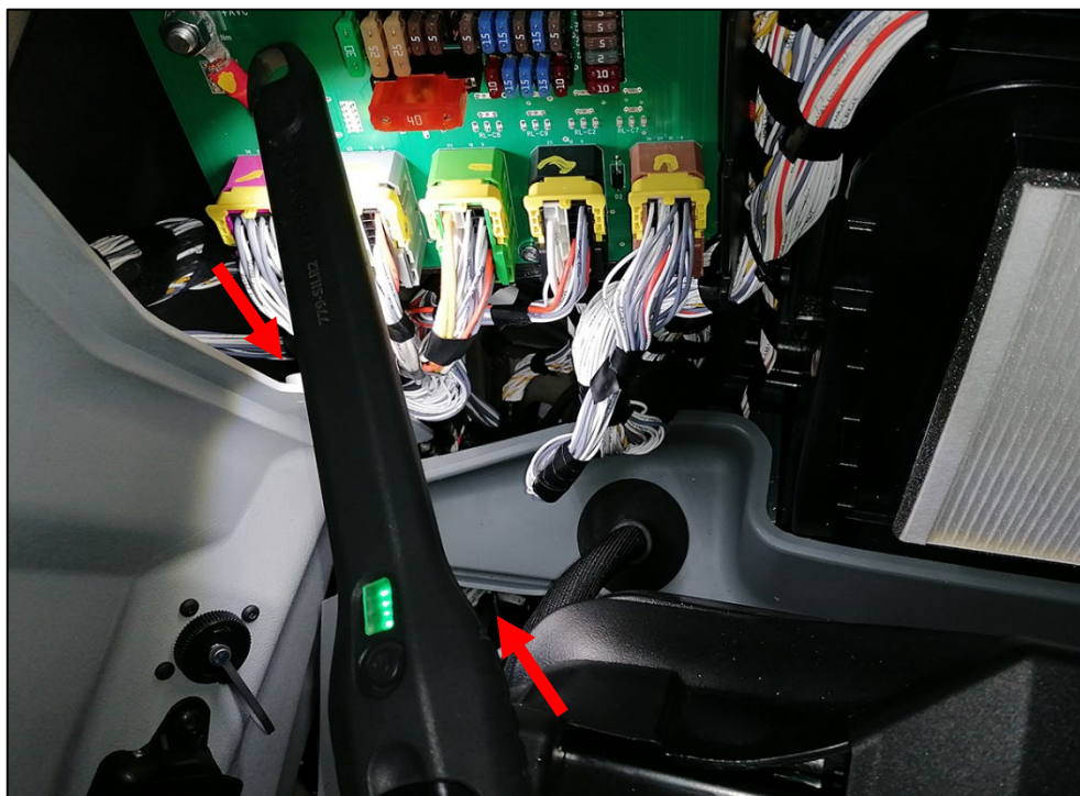
Plugue para o prensa-cabo: vista de dentro da cabine na parte de trás à direita
